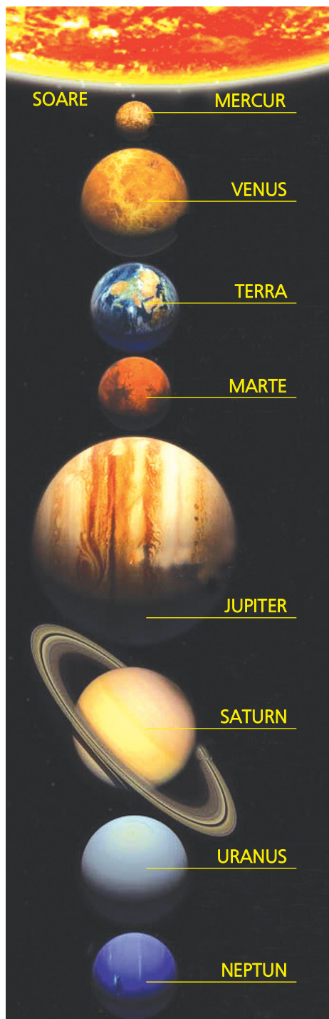
Sistemul Solar
