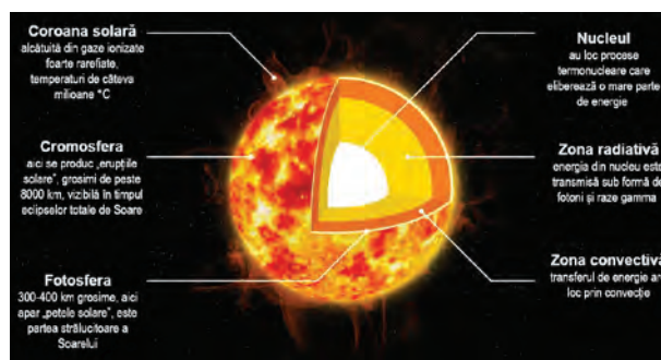
Fig. 3 Structura Soarelui: interior și atmosferă solară.
