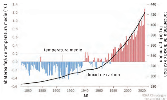
Fig. 2 Corelația dintre evoluția temperaturilor medii globale și evoluția cantității de dioxid de carbon eliminat de oameni în atmosferă, 1850–2024.
