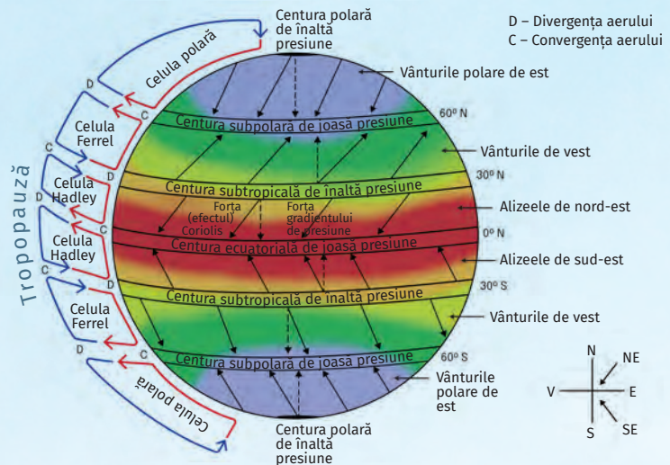
Fig. 7 Zonele de căldură și distribuția spațială a zonelor de presiune atmosferică și a vânturilor permanente
