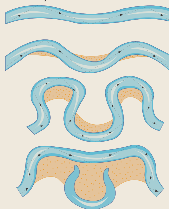
Fig. 2 Formarea meandrelor.
