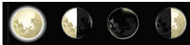
Fig. 4 Fazele principale ale Lunii: 1) Lună Plină, 2) Ultimul Pătrar, 3) Lună Nouă, 4) Primul Pătrar.
