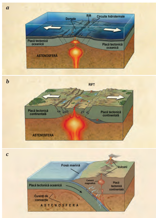
Fig.2 Tipuri de contact tectonic: rift în bazine oceanice (a), rift pe uscat (b), zonă de subducție (c).
