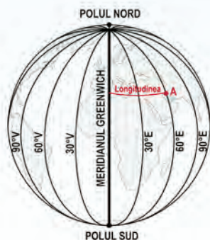
Fig. 2 Meridiane care indică distanța măsurată în grade față de meridianul de zero grade, Greenwich.
